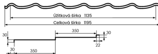
Technický nárys
